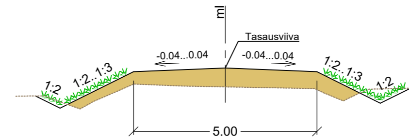
Y11, Y12 ja Y16 peruspoikkileikkaus
