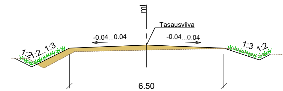
Y7 peruspoikkileikkaus
