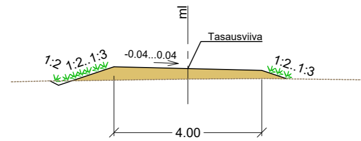
Y10 ja Y14 peruspoikkileikkaus
