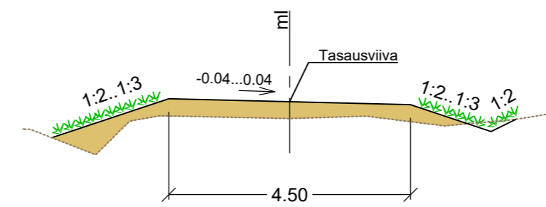
Y4 ja Y15 peruspoikkileikkaus
