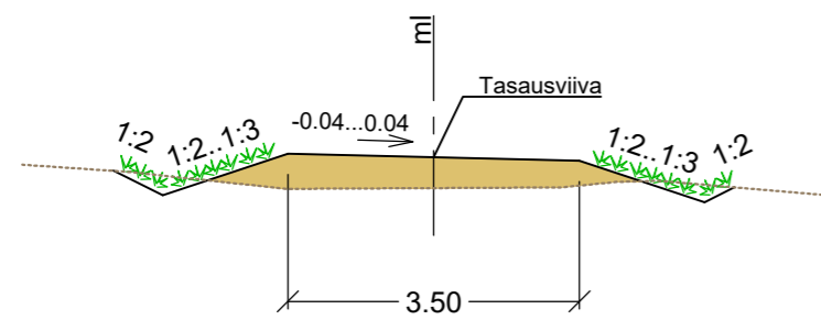
Y1, Y3, Y5, Y6, Y13 ja Y14 peruspoikkileikkaus
