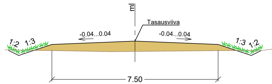
Y8 peruspoikkileikkaus
