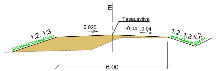
Y2 ja Y9 peruspoikkileikkaus
